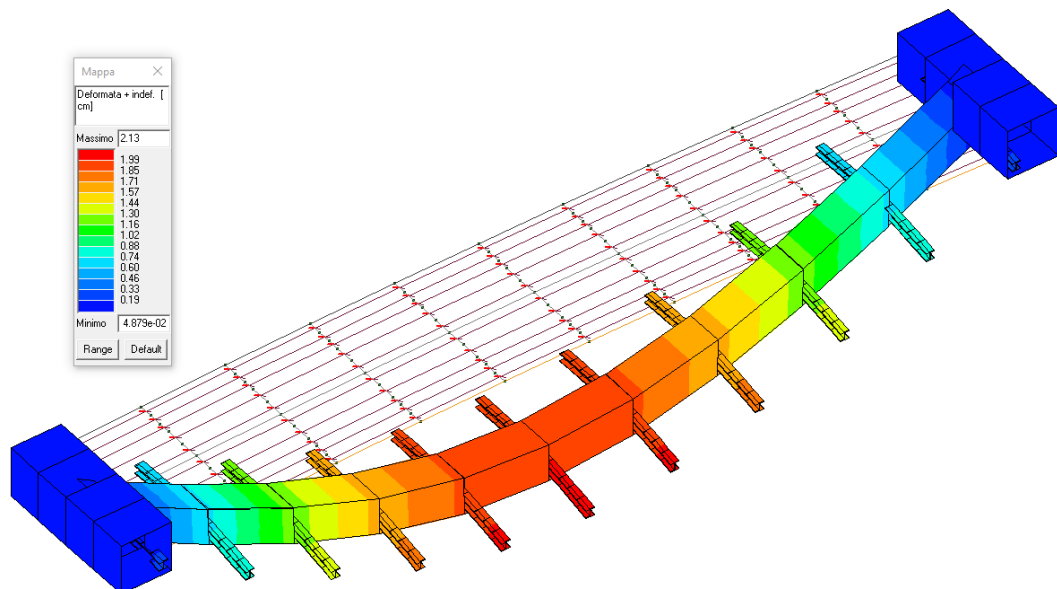
MASSIMA DEFORMATA IN CONDIZIONI STATICHE CON CARICO ESTERNO
