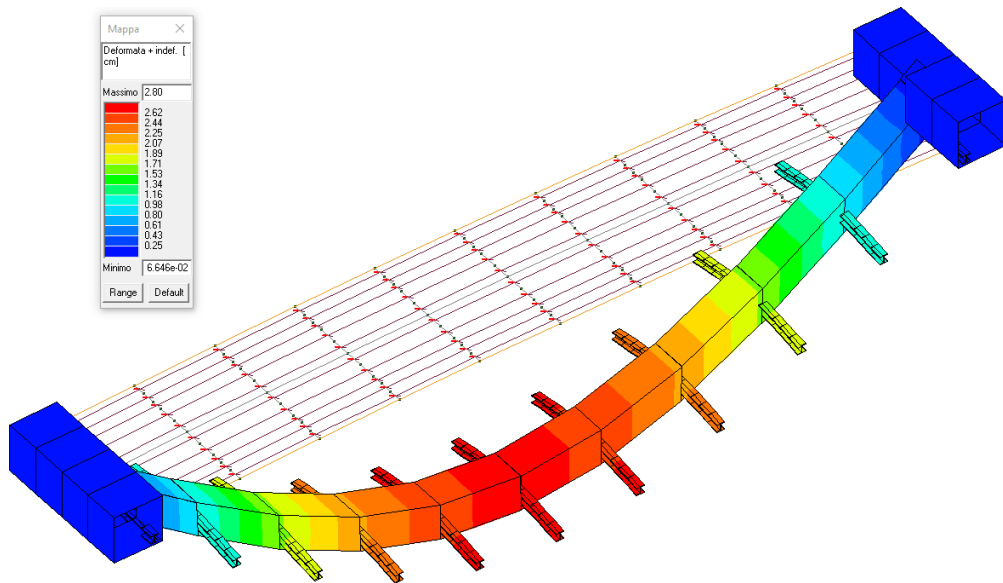
MASSIMA DEFORMATA IN CONDIZIONI STATICHE CON CARICO UNIFORME
